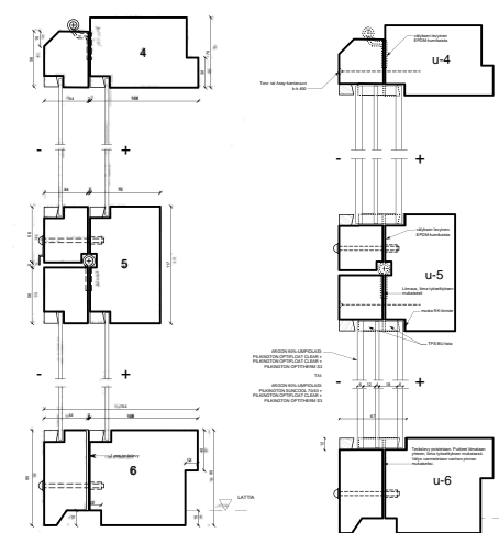
ALKUPERÄINEN URAKKAPIIRUSTUS: Päästäis no 78. Ikkunadetaileja 1/1 (kuvassa 2,5)
