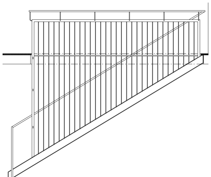
uusi sisäporras P3 1/50
