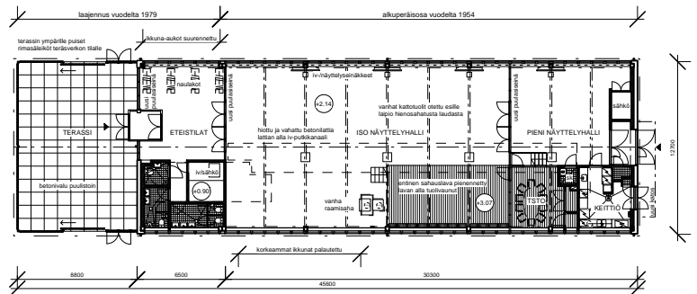
1.krs pohjapiirros 1/500
